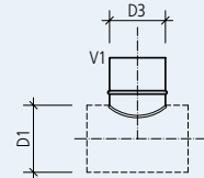
PSV/PSU Sattelstück
