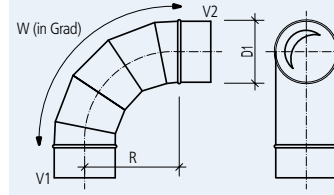
BF/BFU Segmentbogen
