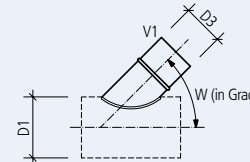
PSV/PSVU Sattelstück mit Winkel
