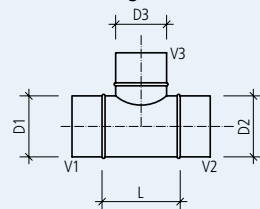
TCP/TCPU Abzweiger 90°
