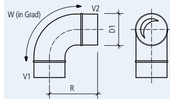
B/BU Bogen gepresst
