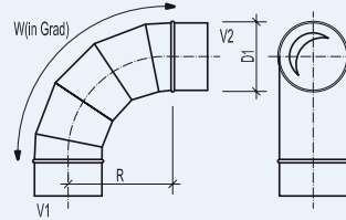
BF/BFU Segmentbogen
