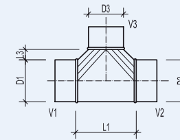
TC/TCU Abzweiger 90°
