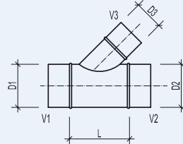
TV/TVU Abzweiger mit Winkel
