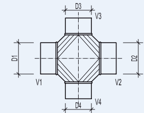
XCP/XCPU Kreuzstück 90°
