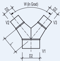
YV/YVU Hosenrohr
