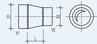
RCL/RCLU Reduktion zentrisch
