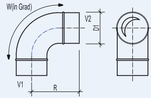
B/BU Bogen gepresst
