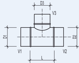
TCP/TCPU Abzweiger 90°
