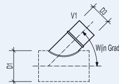
PSV/PSVU Sattelstück mit Winkel
