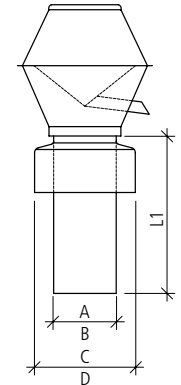
Regenhut eckig mit Regenkragen
