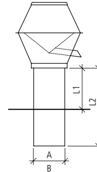
Regenhut eckig mit Tablett (Flachdach 0°)
