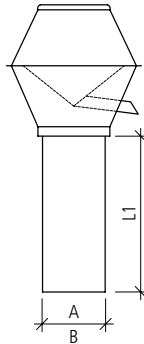
Regenhut eckig mit Standrohr
